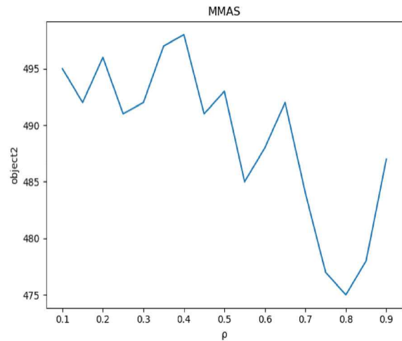
(d) MMAS algorithm parameter selection
